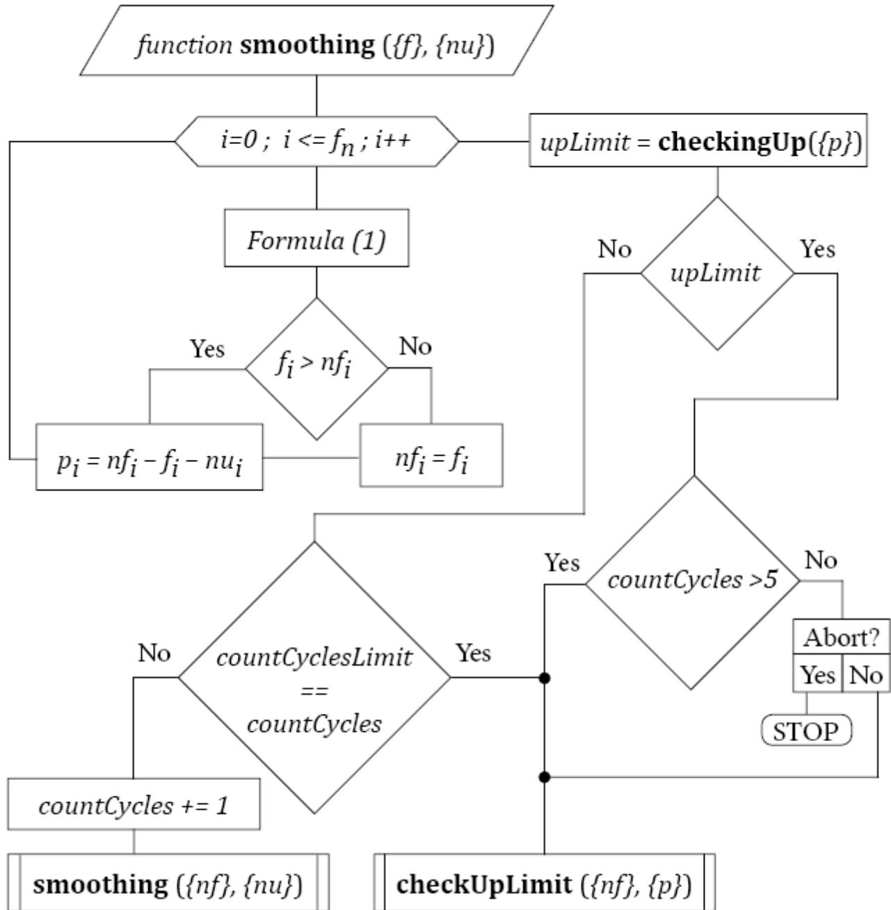
Рис.3 — Схема алгоритму згладжування виміряних вертикальних стріл (функція smoothing ( \{f\}, \{nu\} )); Formula (1) — поліном згладжування по п'яти точках (1); checkingUp ( \{p\} ) — функція перевірки «чистих» підйомок; checkUpLimit ( \{nf\}, \{p\} ) — функція перевірки достатності підйомки для забезпечення розрахункового підвищення.
